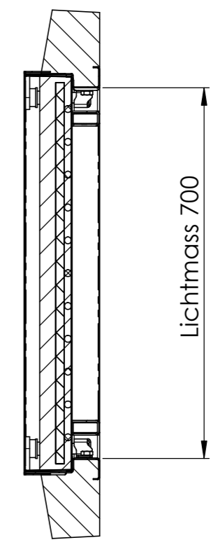
SCHNITT B-B
